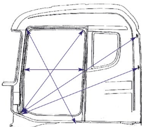
► Control dimensional del lateral de la cabina
